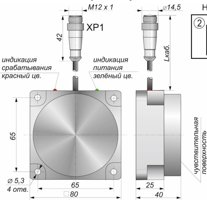
Габаритный чертеж
