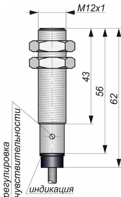
Габаритный чертеж
