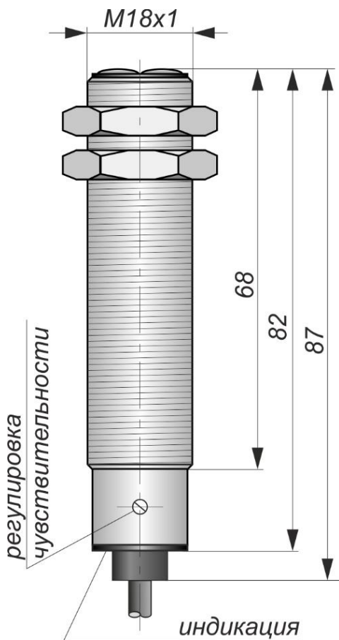
Габаритный чертеж
