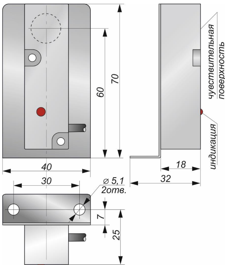
Габаритный чертеж
